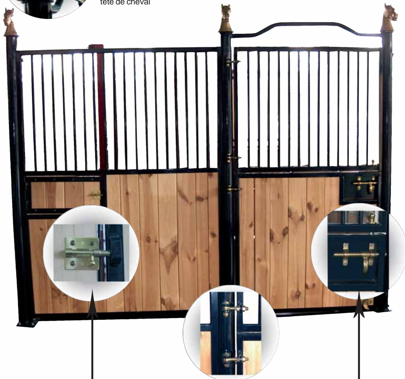
Portillon pour mangeoire
